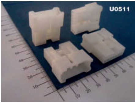
12 P M, RT C-90, Ny-66
